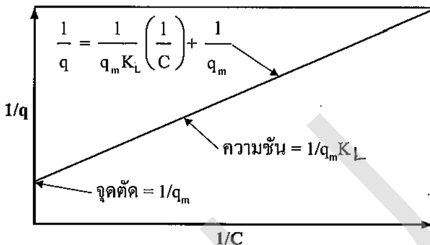
ภาพที่ 2-3 ไอโซเทอร์มการดูดซับแบบเชิงเส้นของแลงเมียร์
