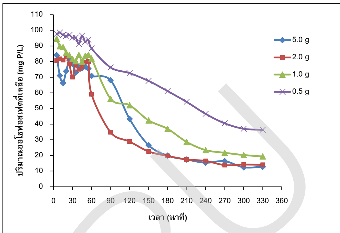
ภาพที่ 4-2 ปริมาณออร์โธฟอสเฟตในน้ำตัวอย่างสังเคราะห์หลังการดูดซับด้วย \text{CaCO}_3 จากเปลือกไข่ที่ปริมาณต่างๆ เวลาในการดูดซับตั้งแต่ 5-330 นาที
