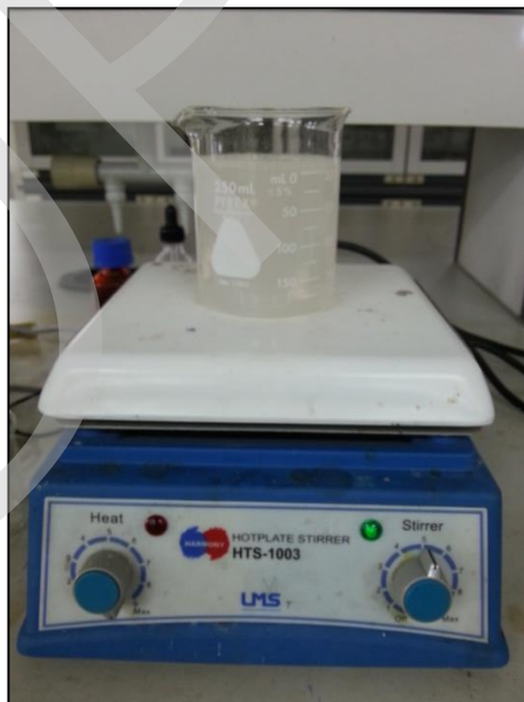
ภาพที่ ค-2 เครื่อง HTS 1003 Hotplate Magnetic Stirrer บริษัท LMS Company (Japan)
