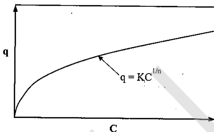
ภาพที่ 2-5 ไอโซเทอร์มการดูดซับแบบไม่เชิงเส้นของฟรอนด์ซ
