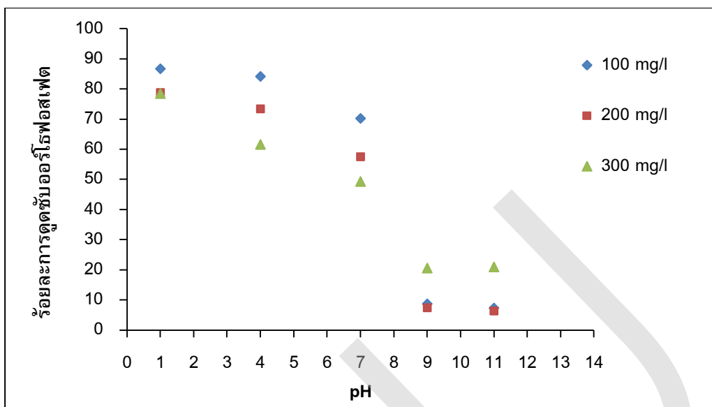
ภาพที่ 4-8 ร้อยละการดูดซับออร์โธฟอสเฟตในน้ำตัวอย่างสังเคราะห์ที่ pH ต่างๆ ด้วยแคลเซียมคาร์บอเนตจากเปลือกไข่ 2.0 g โดยใช้เวลาในการดูดซับ 180 นาที
