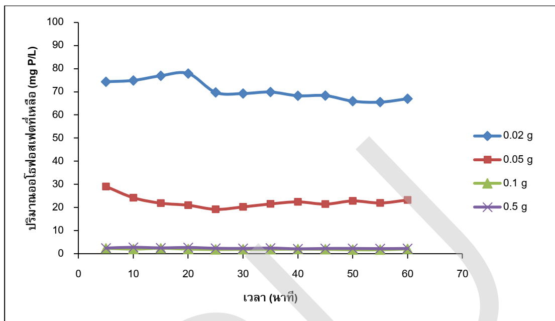
ภาพที่ 4-4 ปริมาณออร์โธฟอสเฟตในน้ำตัวอย่างสังเคราะห์หลังการดูดซับด้วยแคลเซียมออกไซด์จากเปลือกไข่เผาในปริมาณต่างๆ เวลาในการดูดซับตั้งแต่ 5-60 นาที
