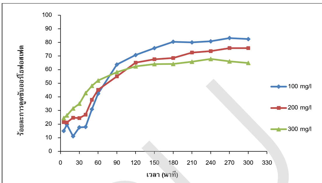
ภาพที่ 4-6 ร้อยละการดูดซับออร์โทฟอสเฟตในน้ำตัวอย่างสังเคราะห์ด้วยแคลเซียมคาร์บอเนตจากเปลือกไข่ 2.0 g โดยใช้เวลาในการดูดซับ 5-300 นาที
