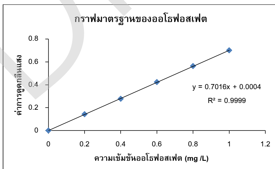
ภาพที่ ก-1 แสดงกราฟมาตรฐานความสัมพันธ์ระหว่างความเข้มข้นของออร์โธฟอสเฟตกับค่าการดูดกลืนแสง
