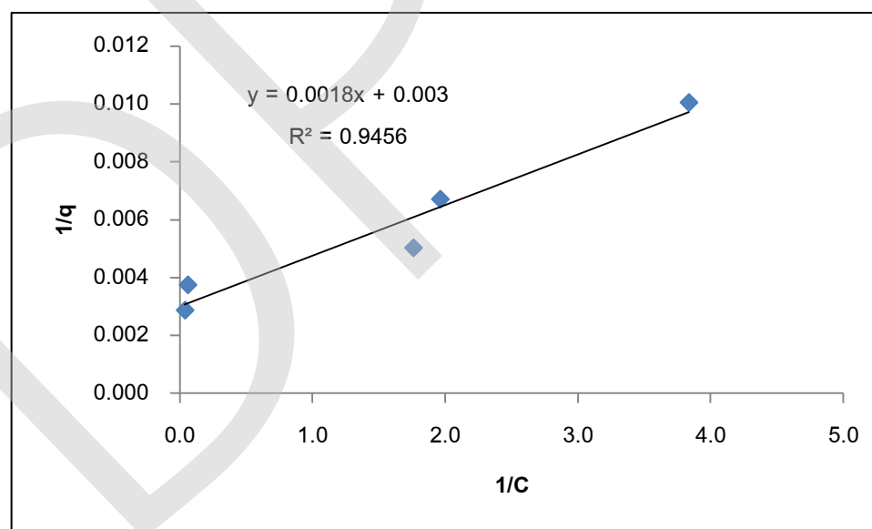
ภาพที่ 4-13 แลงเมียร์ไอโซเทอร์มของการดูดซับออร์โทฟอสเฟตด้วย \text{CaO} จากเปลือกไข่เผา ที่ pH เท่ากับ 11
