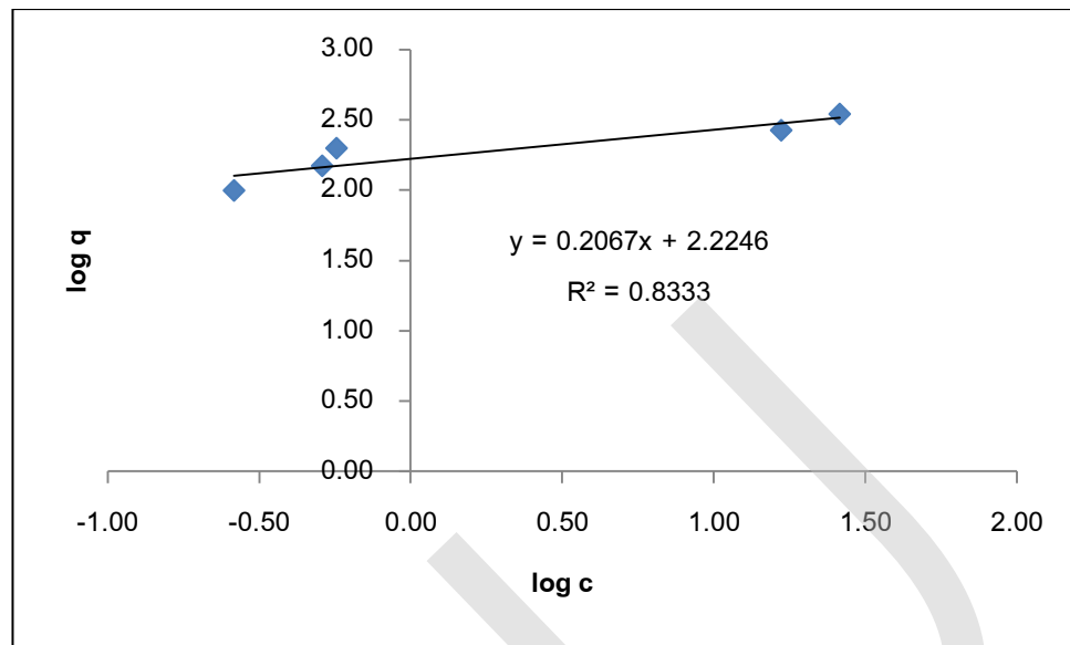
ภาพที่ 4-11 ฟรอนดิชไอโซเทอร์มของการดูดซับออร์โธฟอสเฟตด้วย CaO จากเปลือกไข่เผา ที่ pH เท่ากับ 11
