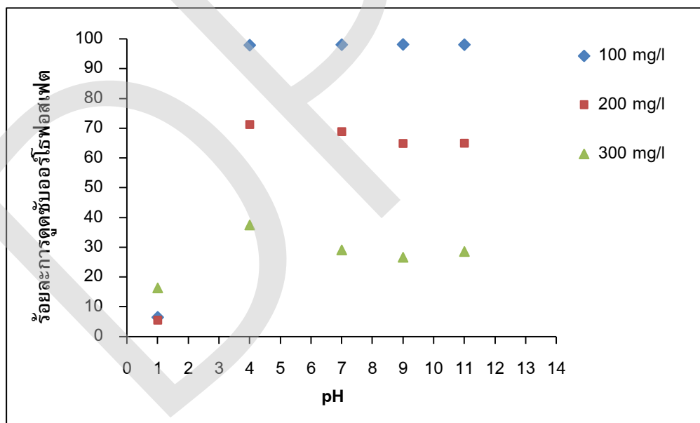
ภาพที่ 4-9 ร้อยละการดูดซับออร์โธฟอสเฟตในน้ำตัวอย่างสังเคราะห์ที่ pH ต่างๆ ด้วยแคลเซียมออกไซด์จากเปลือกไข่เผา 0.1 g โดยใช้เวลาในการดูดซับ 30 นาที
