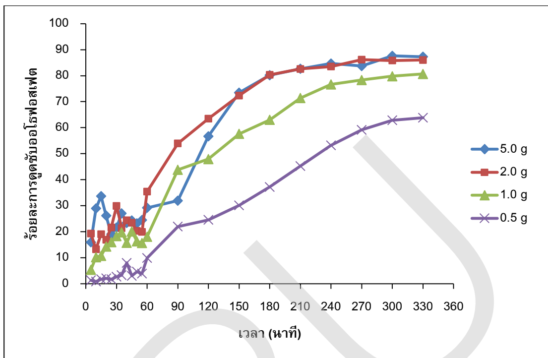
ภาพที่ 4-3 ร้อยละการดูดซับออร์โธฟอสเฟตในน้ำตัวอย่างสังเคราะห์ด้วย \text{CaCO}_3
