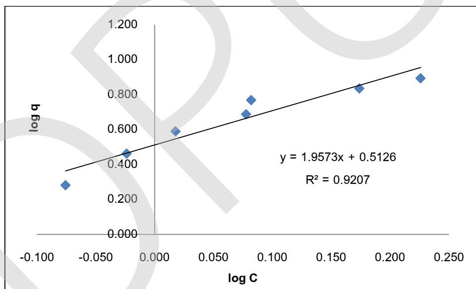
ภาพที่ 4-10 ฟรอนดิชไอโซเทอร์มของการดูดซับออร์โทฟอสเฟตด้วย \text{CaCO}_3 จากเปลือกไข่ที่ pH เท่ากับ 1
