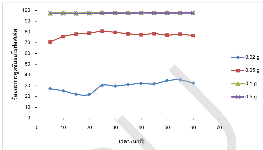
ภาพที่ 4-5 ร้อยละการดูดซับออร์โธฟอสเฟตในน้ำตัวอย่างสังเคราะห์ด้วยแคลเซียมออกไซด์จากเปลือกไข่เผาที่ปริมาณต่างๆ โดยใช้เวลาในการดูดซับ 5-60 นาที
