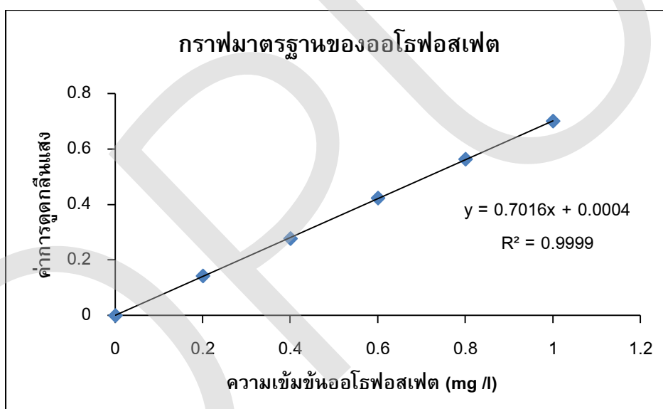
ภาพที่ 4-1 กราฟมาตรฐานความสัมพันธ์ระหว่างความเข้มข้นของออร์โธฟอสเฟตกับค่าการดูดกลืนแสง
